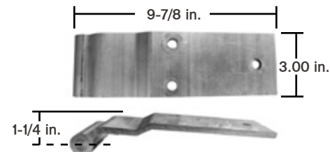
Swing Door Hinge, 3-Hole Material: Aluminum
