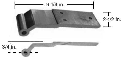
Swing Door Hinge, 3-Hole Material: Aluminum
