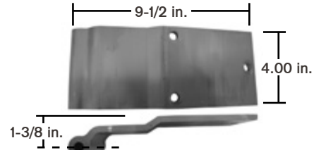
Swing Door Hinge, 3-Hole Material: Aluminum
