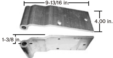
Swing Door Hinge, 3-Hole Material: Aluminum
