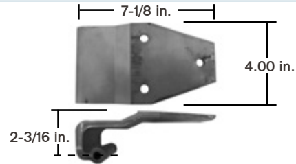
Swing Door Hinge, 3-Hole Material: Aluminum
