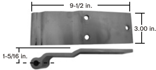
Swing Door Hinge, 3-Hole Material: Aluminum
