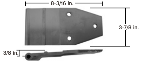
Swing Door Hinge, 3-Hole Material: Aluminum
