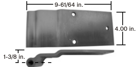
Swing Door Hinge, 3-Hole Material: Aluminum
