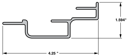
Side Door Header New GVSD
