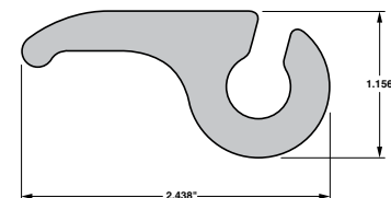
Side Door Lock Rod
